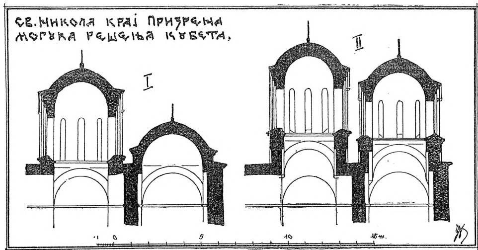
Сл. 2. — Две могућности решења кубета Св. Николе.
